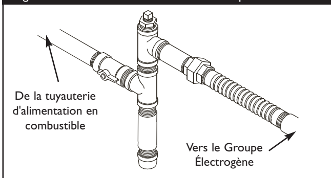
Figure 34 — Raccords de Combustible Complétés
